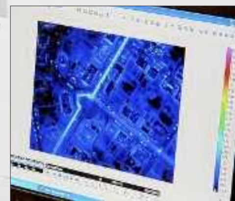
L'avenue Passaga, à Forbach, sujette à des déperditions de chaleur.
