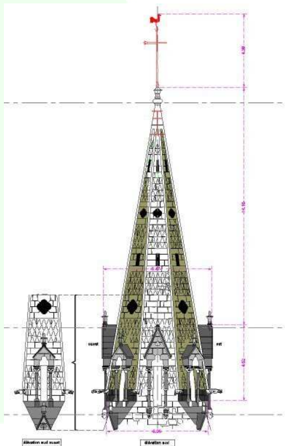
Relevé 1/10 ème de la flèche de l'Eglise Saint-Remy de Forbach pour reconstruction à l'identique
